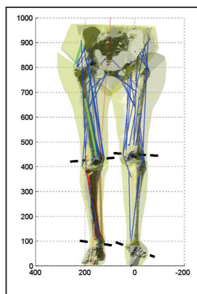
Modello muscoloscheletrico degli arti inferiori. Il modello si riferisce ad uno specifico paziente di cui erano disponibili dati di tomografia computerizzata (CT), risonanza magnetica (MR) e analisi del movimento. Il modello consente di calcolare le forze espresse dai muscoli e agenti sulle ossa in ogni istante del movimento.
